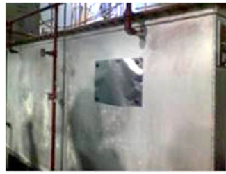
遮熱シート サンプル 貼付中
